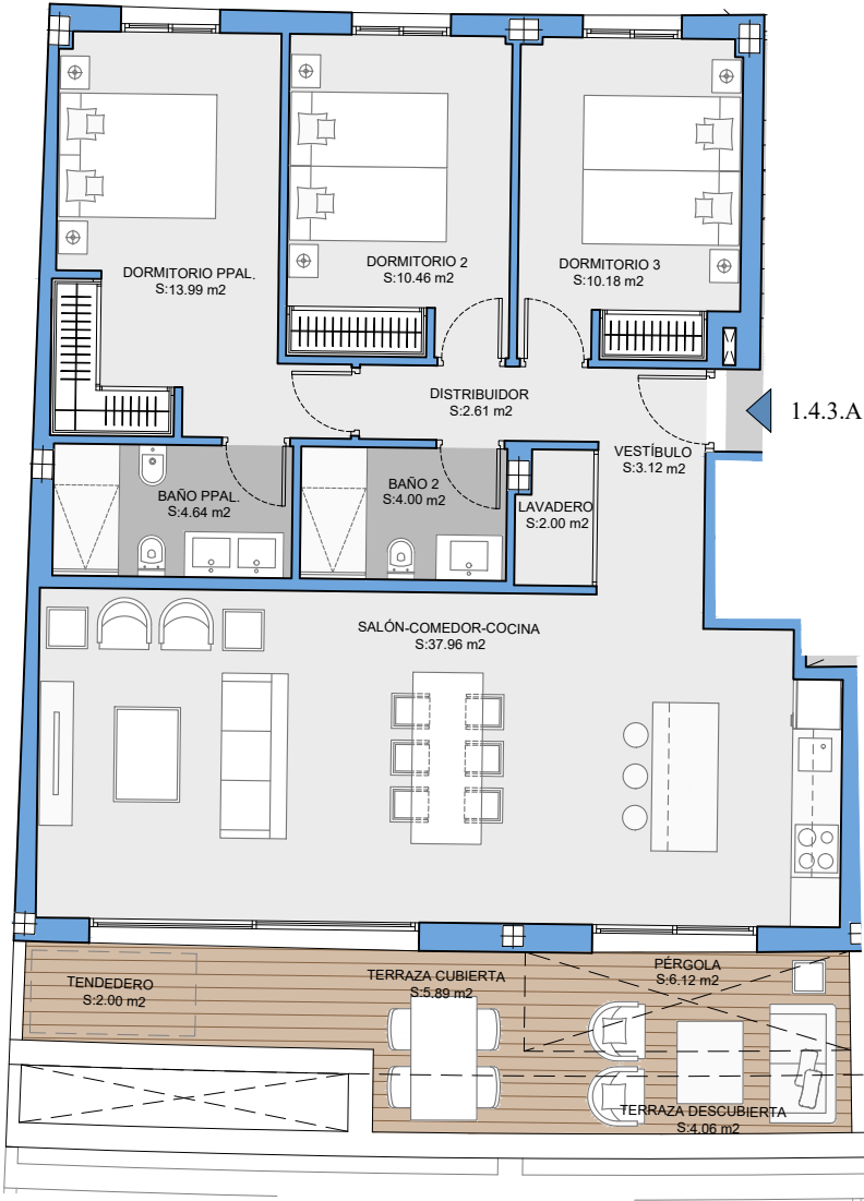
PLANTA SEGUNDA
